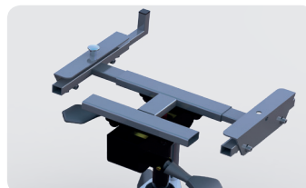
Croix de fixation rapide pour plateau avec butée arrière et doigt d'indexage
